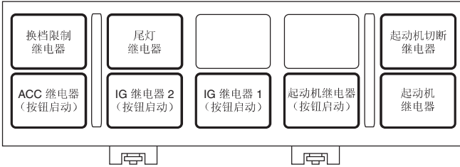
继电器支架 (2.5 L 涡轮增压车型, 3.6 L 车型)
