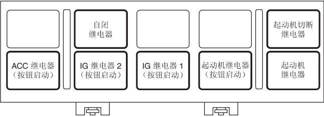
继电器支架 (2.0 L 和 2.5 L 非涡轮增压车型 (发动机型号 FB), 2.5 L 非涡轮增压车型 (发动机型号 EJ))
