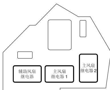
空调继电器支架 (2.0 L 和 2.5 L 非涡轮增压车型 (发动机型号 FB), 2.5 L 非涡轮增压车型 (发动机型号 EJ), 2.5 L 涡轮增压车型)
